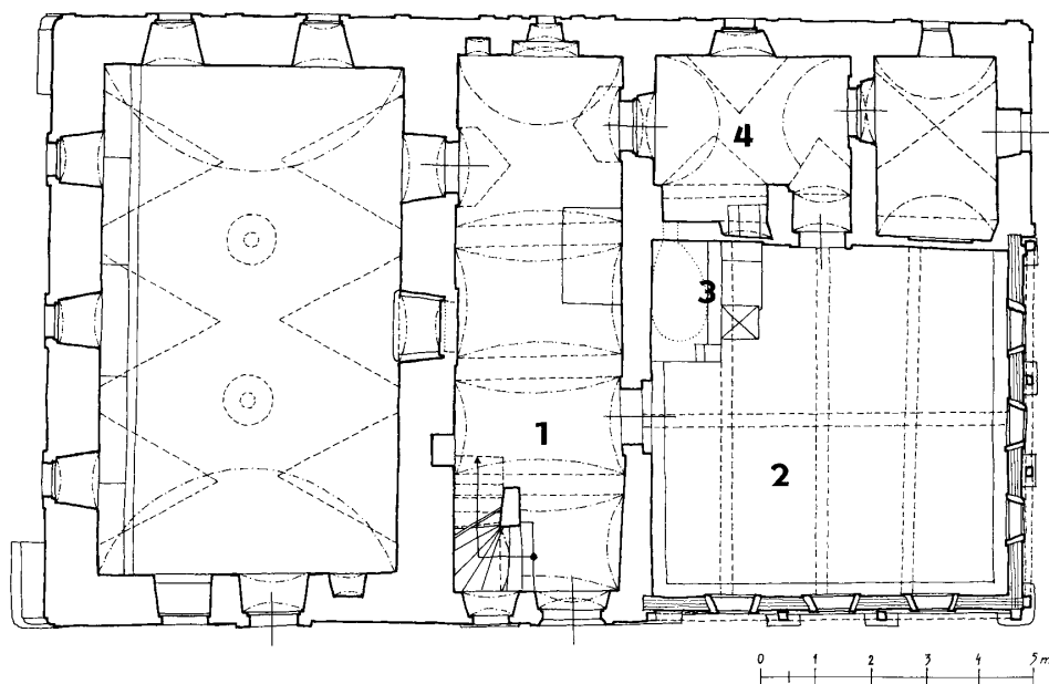
Obr. 4: Půdorys přízemí domu čp. 12 v Malé Skále (okr. Jablonec nad Nisou) z počátku 19. století jako příklad dispozice s volnou síní a s kuchyní, přesunutou ze síně do druhého traktu vedle světnice. Síní v tomto případě není kvůli místním podmínkám funkčně průchozí a dispozice je chlévního typu s komorami v patře. 1 - síní, 2 - světnice, 3 - topeniště, 4 - kuchyně. (Kresba K. Fousková, 1996.)
