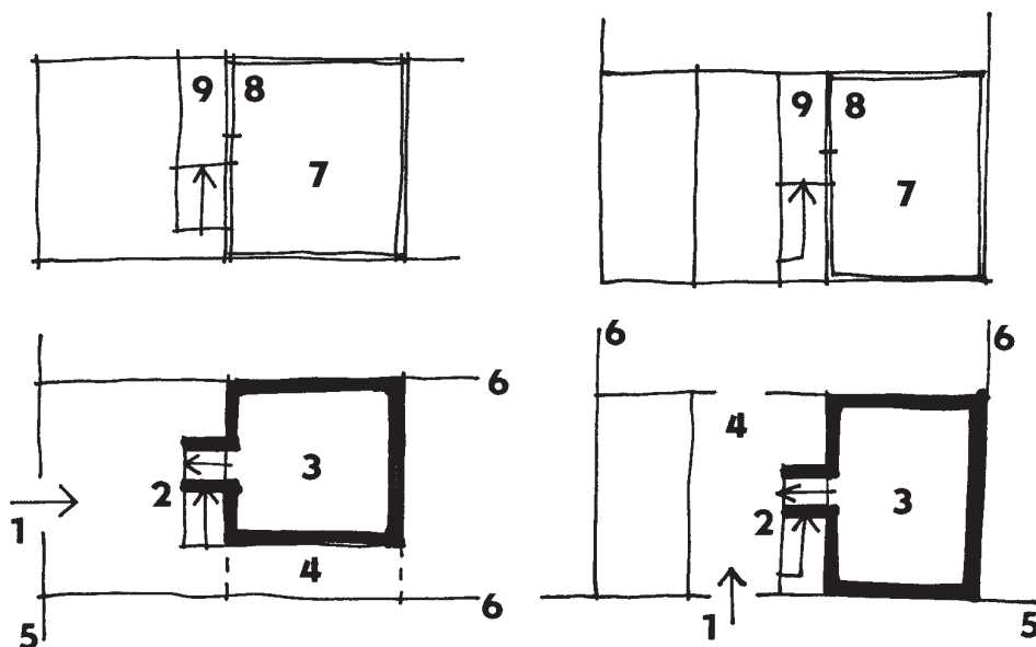
Obr. 1: Srovnávací schemata obvyklého uspořádání síňového domu (vlevo podle M. Radové a M. Hauserové, doplněno) a předpokládaného archetypu domu čp. 15 v Zelenářské ulici ve Znojmě. 1 - vstup, resp. vjezd, z ulice, 2 - aparát šijového sestupu do spodní zděné komory a peronového výstupu k obytné místnosti nad komorou, 3 - zděná komora, 4 - chodba, resp. průjezd ke dvoru, 5 - uliční čára, 6 - hranice parcel sousedních domů, 7 - roubená obytná místnost nad komorou, 8 - kout s otopným zařízením, při vývoji od jizby ke světnici přecházející k nepřímému vytápění z konce peronu (9). (Kresba autor, 1996.)
