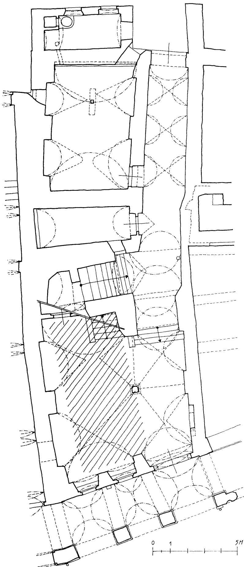
Obr. 7: Příklad typického půdorysu městského domu s velkou renesančně klenutou síní, s průjezdem na dvůr kolem gotické zděné komory. Ta je dodatečně renesančně zaklenutá, se vstupem z průjezdu, jehož mladší ostění je vloženo do niky původního gotického portálu. Situace (vyšrafováno) gotického sklepa pod síní naznačuje, že archetyp domu mohl být průjezdový a nikoli síňový. Sín reaguje v tomto případě na sklep i umístěním klenbových podpěr, loubí "vykročilo" před starší uliční čáru rovněž až při zděné renesanční přestavbě. Telč (okr. Jihlava) čp. 6, s použitím zaměření J. Lojky. (Kresba K. Fousková, 1996.)
