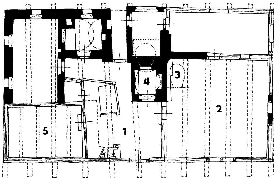
Obr. 3: Půdorys přízemí domu čp. 22 ve Zbečně (okr. Rakovník). Vesnický roubený dům, situovaný nezvykle svou podélnou vstupní stranou do uliční čáry. Středověkého původu, je jeho jednotraktové trojdílné jádro "pravé" orientace s průchozí síní: 1 - síň, 2 - světnice, 3 - středověká pec někdejší dymné jizby, 4 - dochovaná mladší kuchyně v koutu síně, pod zděným komínem, 5 - zbytek dvoupodlažní zadní komorové části domu. (Kresba K. Fousková, 1996.)
