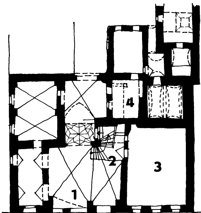
Obr. 2: Půdorys přízemí domu č. 3 ve Velké Mikulášské ulici ve Znojmě podle V. Mencla (Městanský dům českého středověku, ZPP roč. 13, 1953, č. 6, s. 182). Struktura domu, dotvořená v tomto případě velkou přestavbou v polovině 16. století, je v principu velmi podobná domu v Zelenářské ulici. 1 - průjezdová síň, 2 - schodišťový uzel u vstupu do světnice, 3 - světnice, 4 - kuchyně. V kuchyni bylo ještě dochováno dymníkové ústí komína nesené úhlovou sestavou trámů, vyvěšenou kovaným táhlem. Levá užší část domu obsahuje komory v charakteristickém půdorysném odstupu, které poněkud člení střední díl domu na širší síň vpředu a užší zadní část s průjezdem na dvůr. (Kresba autor, 1996.)
