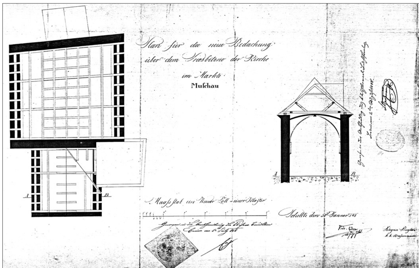
Obr. 9: Mušov, kostel sv. Leonarda, plán na opravu kostela a krovu ze 30. ledna 1848, sign. Peregrin Biegler (MZA Brno).
