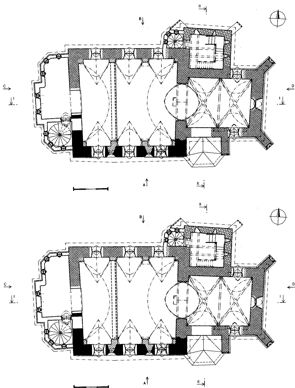
Obr. 3: Mušov, kostel sv. Leonarda, půdorys kostela ve dvou řezových rovinách s vyznačením stavebního vývoje: černé zdivo románské, šikmo křížkované zdivo gotické (1. fáze), přerušované křížkované zdivo gotické (2. fáze), šrafované zdivo barokní, tečkované zdivo z r. 1802, novodobé úpravy nevyznačeny (zaměření IGM s.r.o. Brno).
