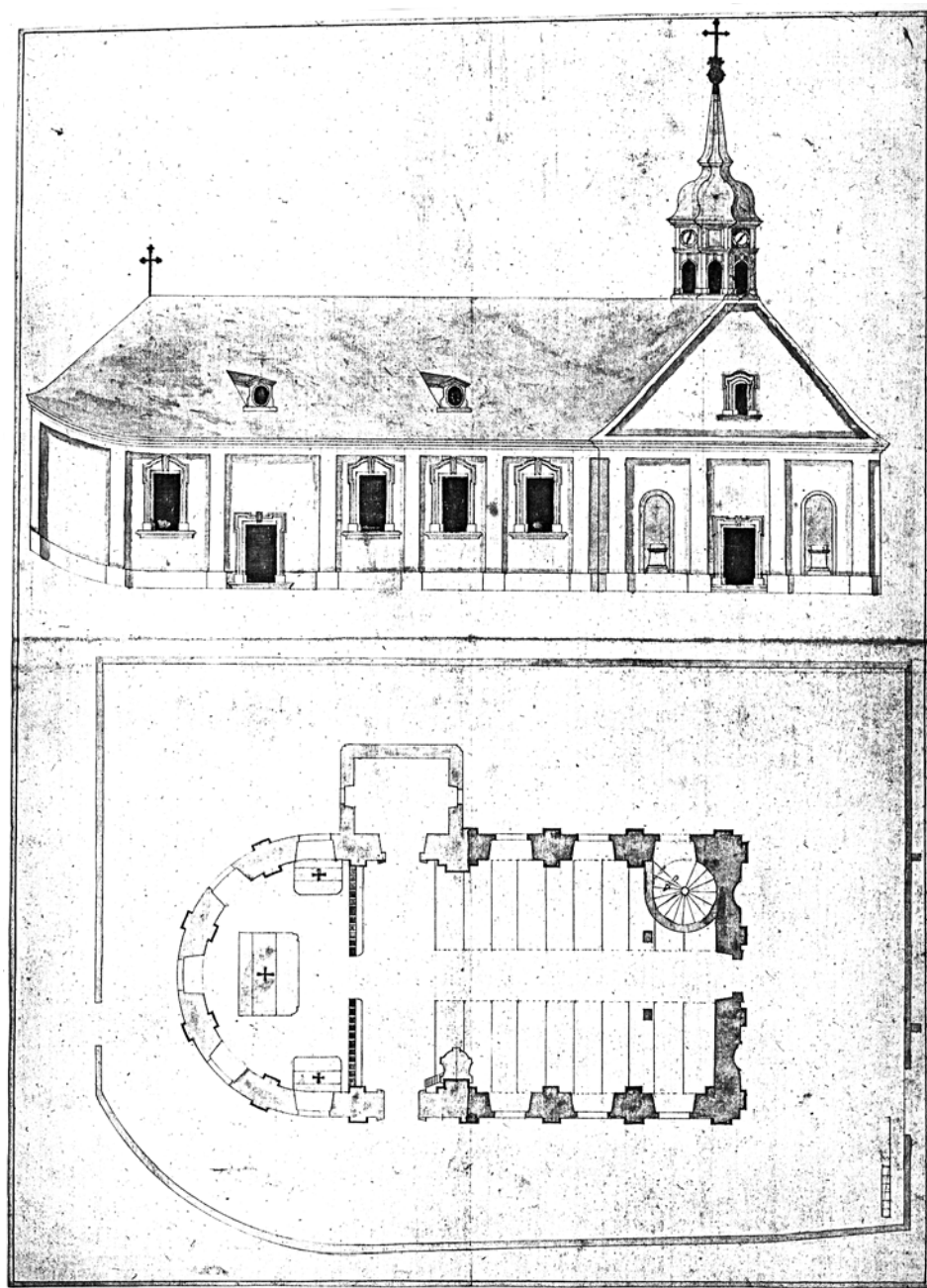
Obr. 6: Mušov, kostel sv. Leonarda, půdorys a nárys nerealizované přestavby kostela, nedat., asi pol. 18. století (MZA Brno).
