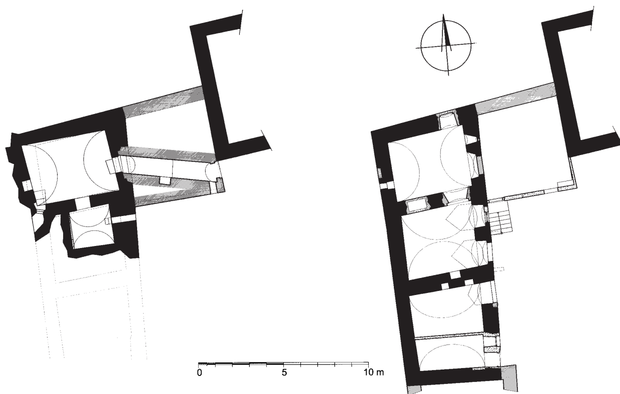
Obr. 21: Černíky, čp. 1. Půdorysy přízemí a sklepa hospodářského objektu ve dvoře usedlosti a západní části obvodového zdiva obytného domu. Tmavě zvýrazněny pozdně středověké konstrukce, šrafovaně pobělohorské, zrnitě recentní (kresba J. Veselý, zaměření J. Kypta a J. Veselý, 2005).
