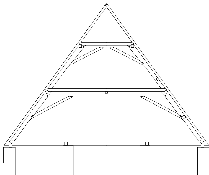
Obr. 14: Pouzdřany, kostel sv. Mikuláše, zaměření krovu lodi, příčný řez plnou vazbou.
