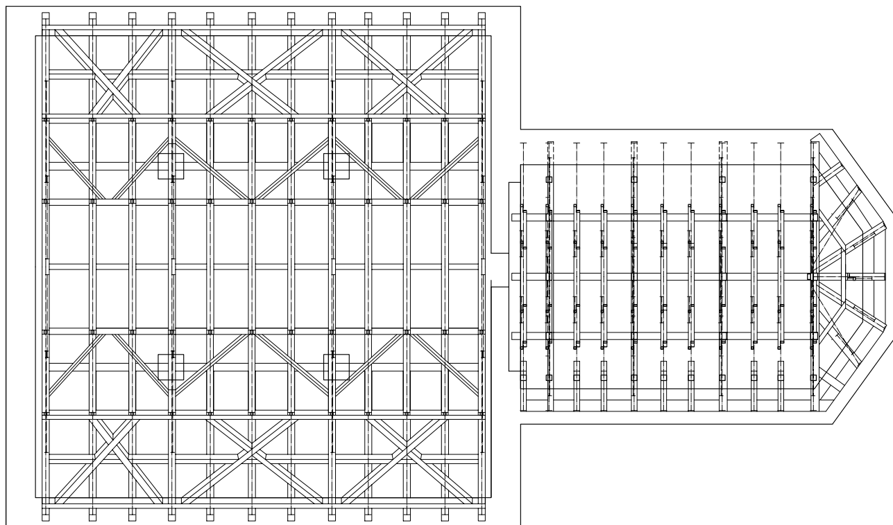
Obr. 13: Pouzdřany, kostel sv. Mikuláše, zaměření krovu lodi a presbytáře, půdorys.
