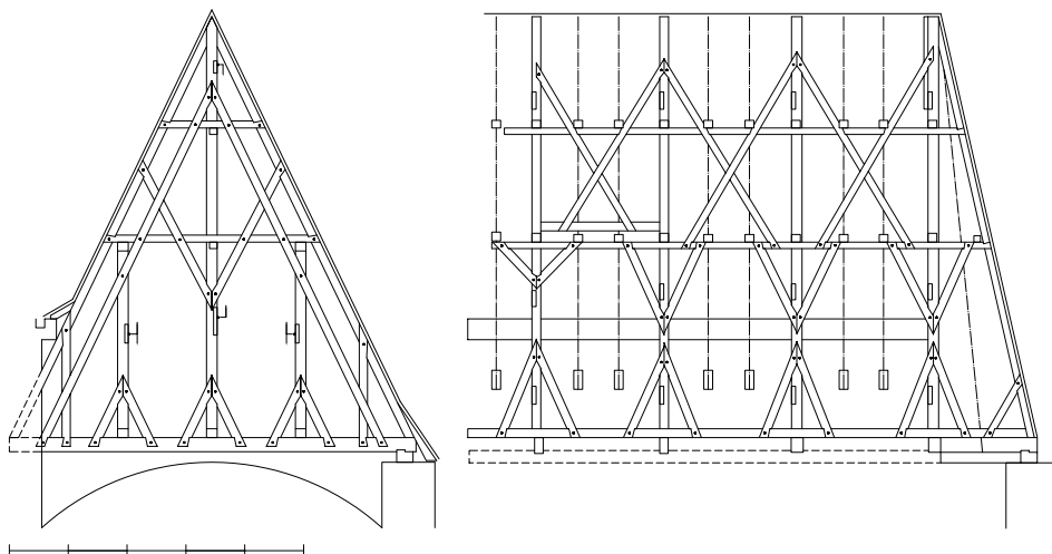
Obr. 12: Pouzdřany, kostel sv. Mikuláše, zaměření krovu presbytáře, příčný a podélný řez (zaměření a kresba obr. 12–15 M. Navrátil, 2013).
