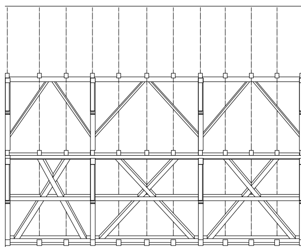
Obr. 15: Pouzdřany, kostel sv. Mikuláše, zaměření krovu lodi, podélný řez.
