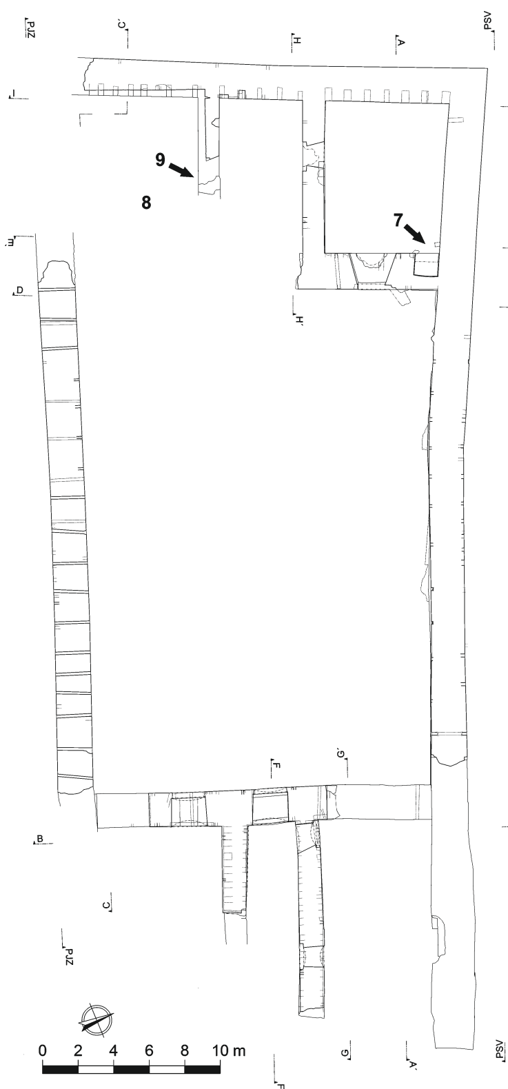
Obr. 16c: Dívčí Kámen, geodetické zaměření půdorysu v úrovni 2. patra (srov. 16a). 7 – zazděný otvor v dolní části krbu (srov. obr. 35–37); 8 – původně vydlážděná místnost (srov. obr. 44); 9 – obslužný otvor kamen ve vydlážděné místnosti (srov. obr. 47).
