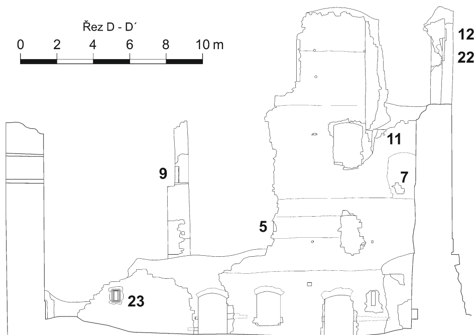
Obr. 31: Dívčí Kámen, geodetické zaměření, pohled od východu na nádvorní průčelí západní obytné části paláce. Vlevo dole okénko s ostěním do přízemí jižního traktu (23). Po stranách řezy oběma spojovacími zdmi (srov. obr. 16a). Rozvedeno u obr. 32.
