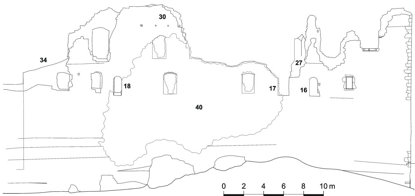
Obr. 63c: Helfenburk, geodetické zaměření severní fasády paláce (srov. obr. 62a). 40 – část fasády porostlá břečťanem.
