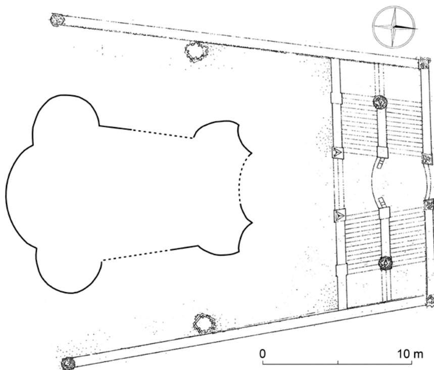
Obr. 11: Smilkov, zámecká zahrada. Spodní část tzv. teatronu s bazénem. Silnou linií vyznačen průběh líce kamenného zdiva bazénu; přerušovanou linií vyznačeny rekonstruované partie (zdívo opěrných zdí a schodiště převzato z plánu z roku 1970, vyhotovila Cupová; zaměření bazénu autoři článku, 2021; úprava plánu F. Laval).
